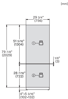
KFMC3632R+L, KFMC3836R+L, KFMC3834R+L, MasterCool III, Ansicht von vorne (*Fußnote) (Skizze)
