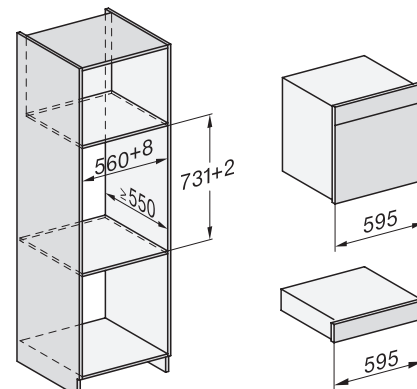
Einbau_DGC_XXL_ESW7x10_EVS7010, Skizze
