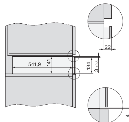
Seitenansicht ESW7x10 EVS7010, Skizze
