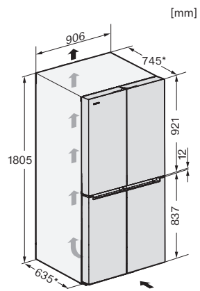
E-Com, KFFD6741 edt/cs, Aufstellskizze
