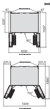
E-Com, KFFD6741 edt/cs, Draufsicht
