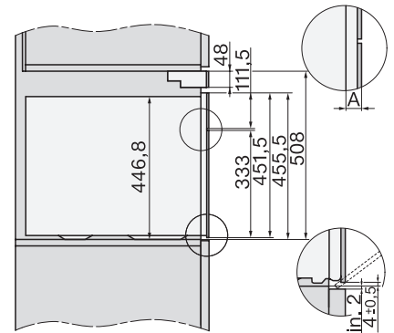
Seitenansicht DGC 7x40-55 Ausgleichsblende oben, Skizze, CH
