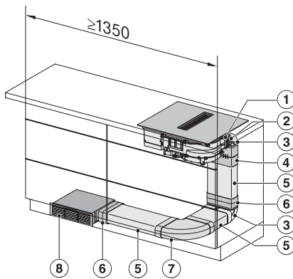
KMDA5649FL, KMDA5649FR, KMDA5649FL MattFinish – Einbauvariante 5 Umluft
