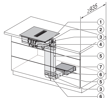
KMDA5649FL, KMDA5649FR, KMDA5649FL MattFinish – Einbauvariante 6 Umluft
