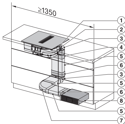
KMDA5649FL, KMDA5649FR, KMDA5649FL MattFinish – Einbauvariante 4 Umluft
