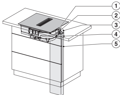
KMDA5649FL, KMDA5649FR, KMDA5649FL MattFinish – Einbauvariante 1 Basis
