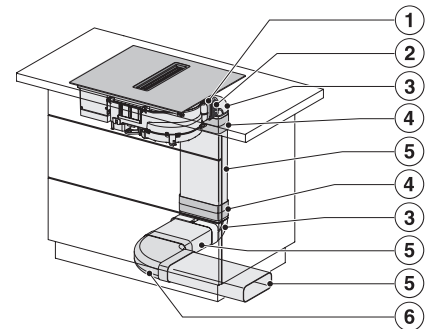
KMDA5649FL, KMDA5649FR, KMDA5649FL MattFinish – Einbauvariante 3 Basis
