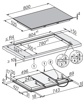
KM8685FL, KM8685FL MattFinish, flächenbündig, (*Fußnote) Skizze
