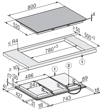
KM8685FL, KM8685FL MattFinish, aufliegender Einbau, (*Fußnote) Skizze
