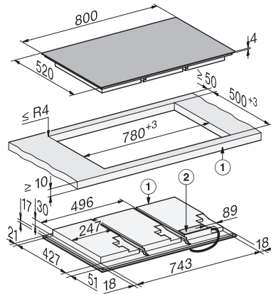
KM8684FL aufliegender Einbau, (*Fußnote) Skizze
