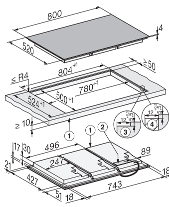
KM8684FL flächenbündig, (*Fußnote) Skizze
