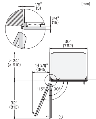
KFMC3632R+L, KFMC3836R+L, KFMC3834R+L, MasterCool III, PACS, mit Edelstahlfront, Draufsicht (Skizze)
