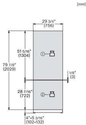
KFMC3632R+L, KFMC3836R+L, KFMC3834R+L, MasterCool III, Ansicht von vorne (*Fußnote) (Skizze)
