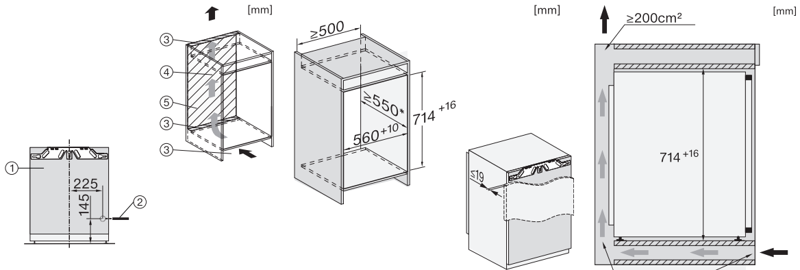
FNS7040E, FNS7040B, FNS7040C, FNS7040D, Installation (*Fußnote) (Skizze)
