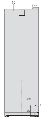
KWT4584E sw, Rioja, Installation (*Fußnote) (Skizze) *1) Ansicht von vorne, 2) Netzanschlussleitung, L = 2200 mm
