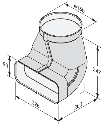
DFK-A90, Adapter, eckig-rund 90°, Skizze
