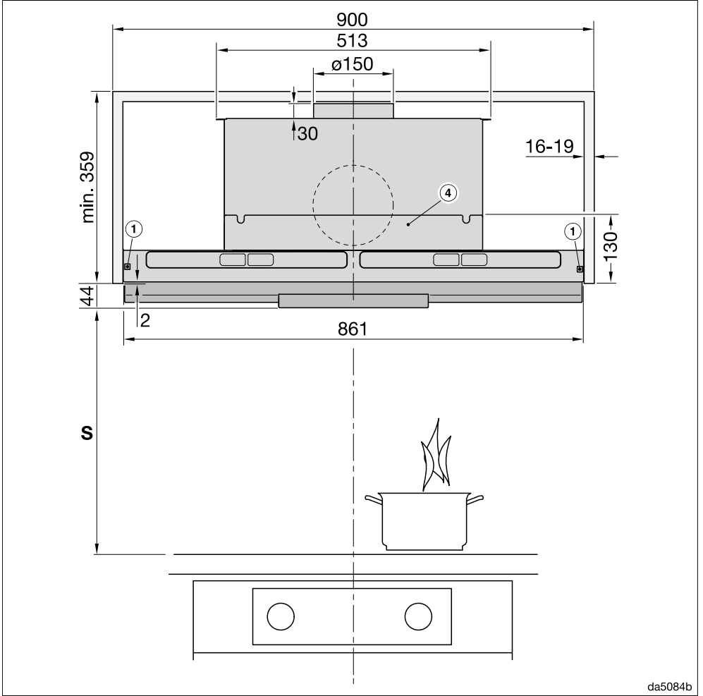
Resim 2: 900 mm genişliğinde bir dolap içinde DAS 8930.
