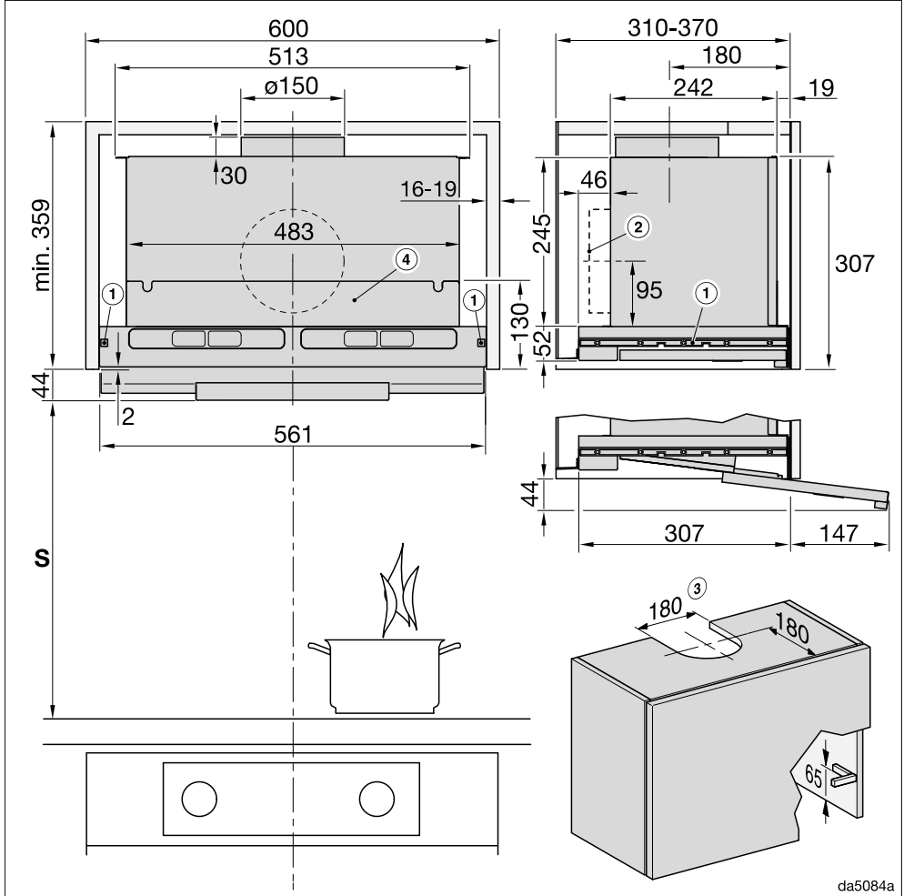
Resim 1: 600 mm genişliğinde bir dolap içinde DAS 8630.
