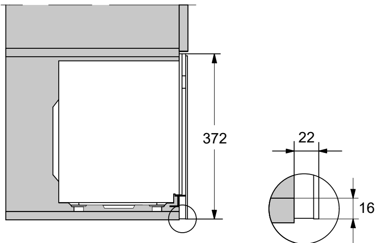
壁柜侧视图
