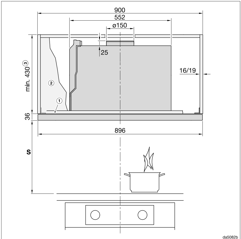
Εικόνα 2: DAS 4931 σε ντουλάπι πλάτους 900 mm.
