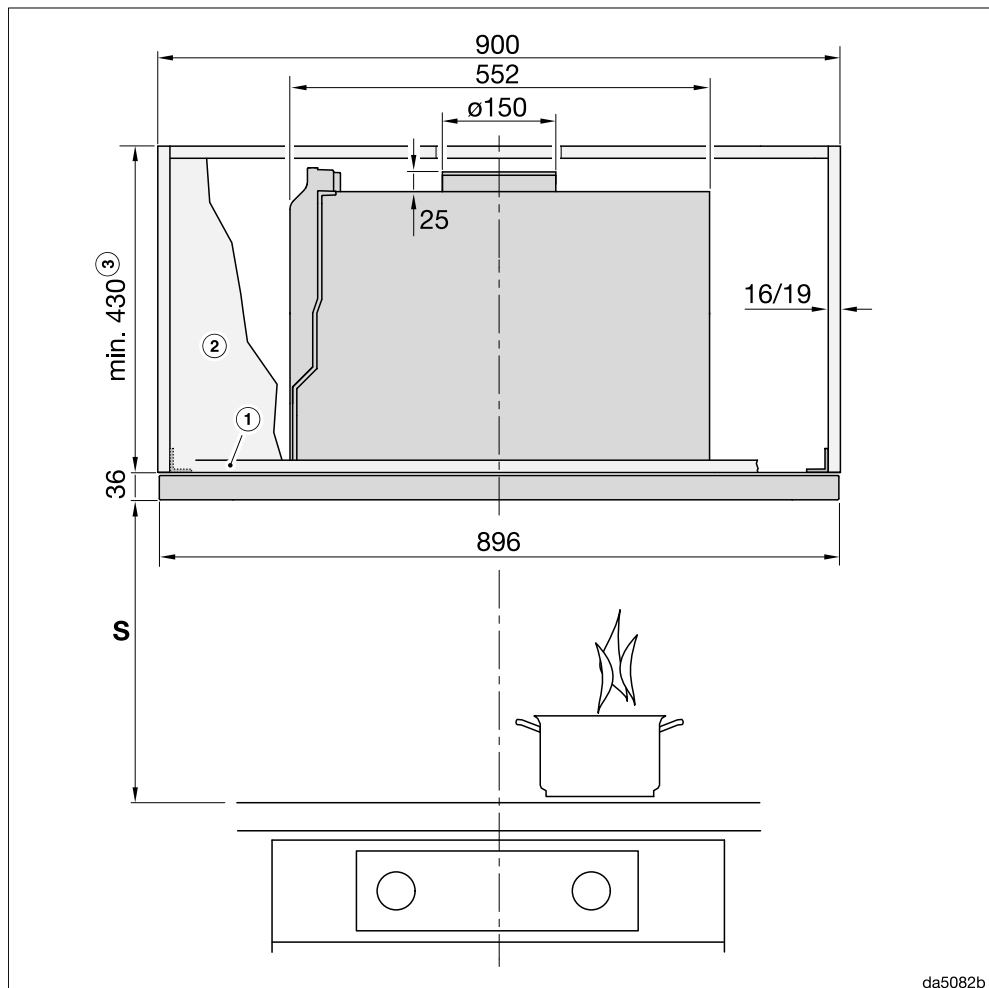
2 pavyzdys: DAS 4931 900 mm pločio spintoje.
