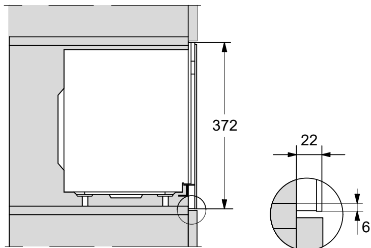
Вид сбоку (высокий шкаф)
