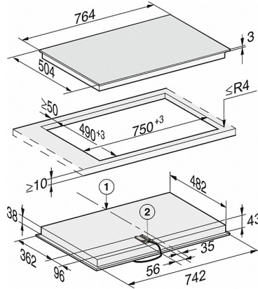
KM 6522 FR, KM 6542 FR (plan d'installation)
