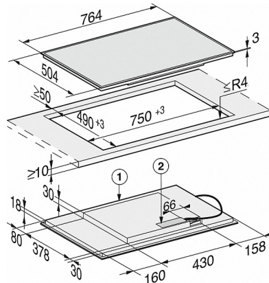
KM 7210 FR, KM 7211 FR (schéma)
