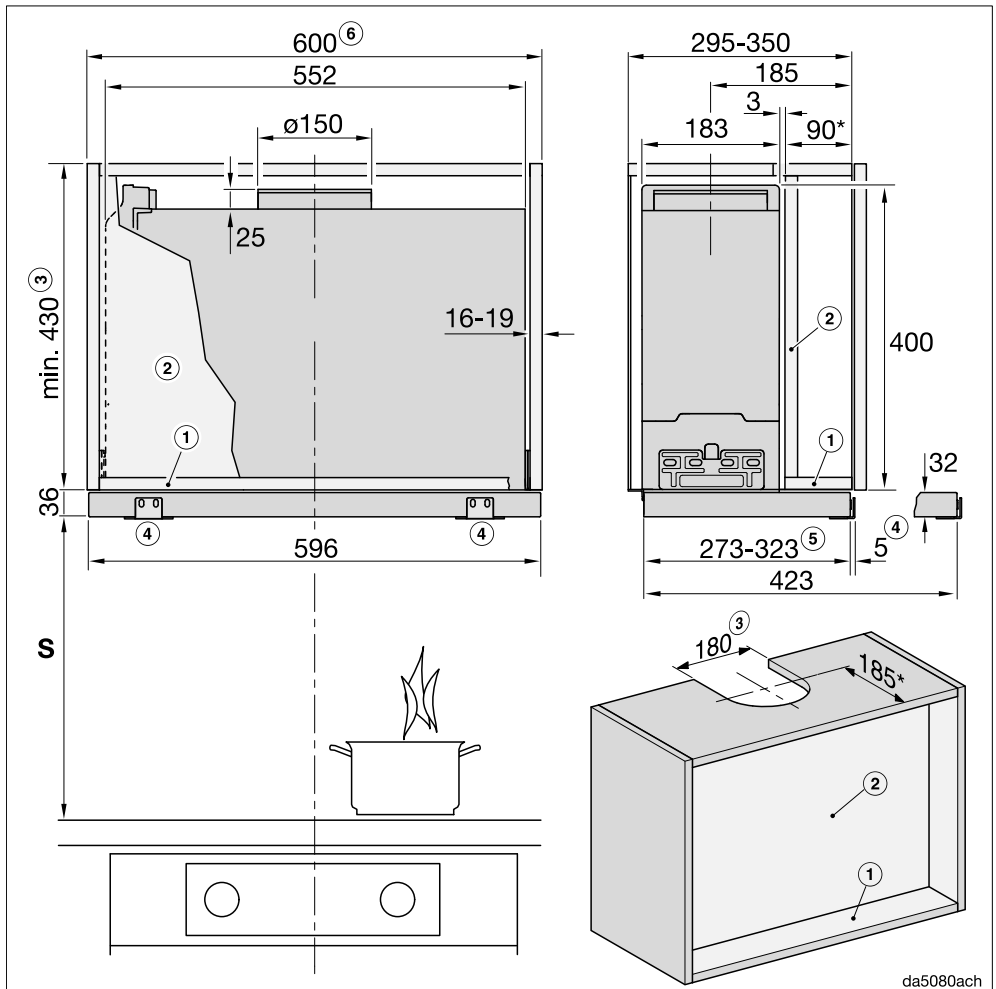
Figura 2: DAS 4620 in un mobile largo 600 mm oppure in una nicchia larga 600 mm
