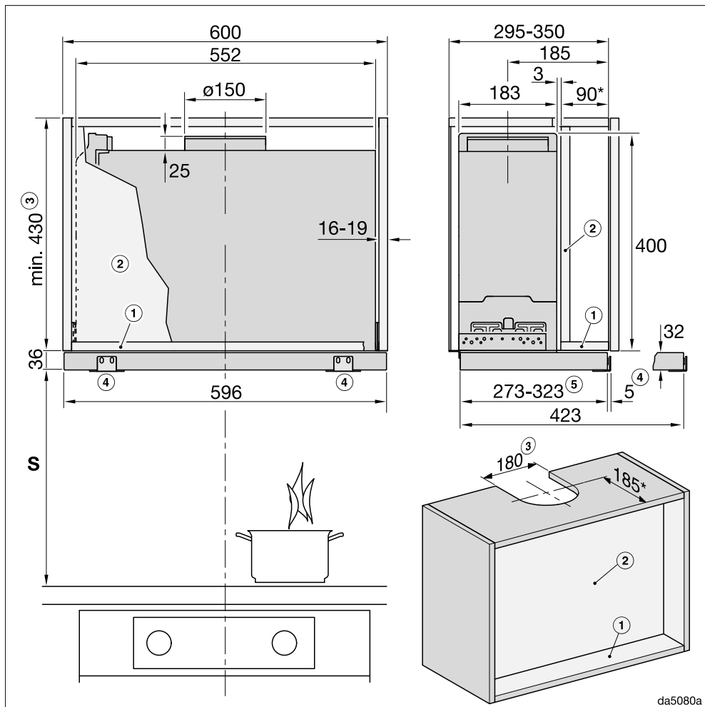
Εικόνα 1: DAS 2620 σε ντουλάπι πλάτους 600 mm.
