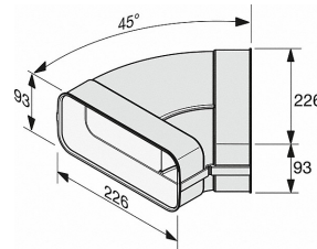
DFK-BH 45, boog, 45° horizontaal, schets
