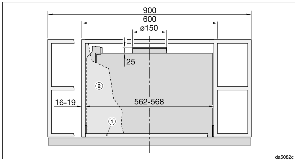
Rysunek 3: DAS 4930 w szafce o szerokości 600 mm lub w szafce o szerokości 900 mm z bocznymi wnękami.
