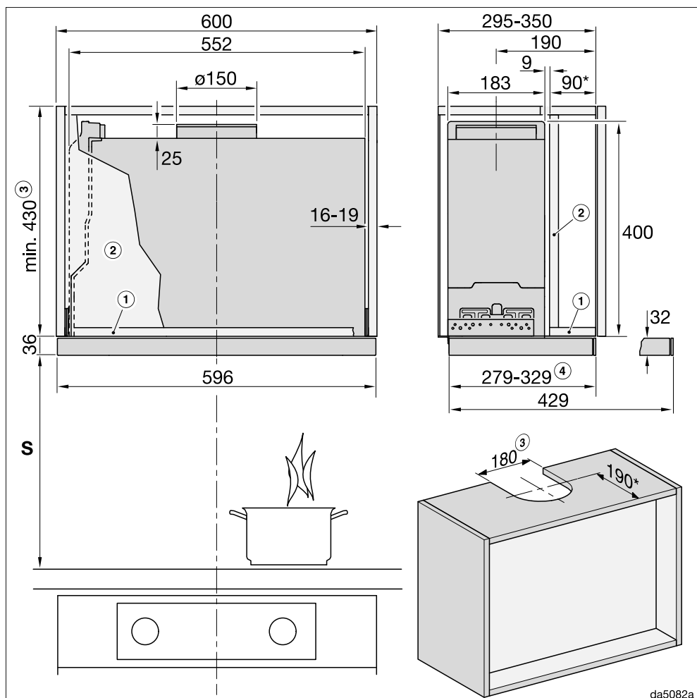
Rysunek 1: DAS 4630 w szafce o szerokości 600 mm.
