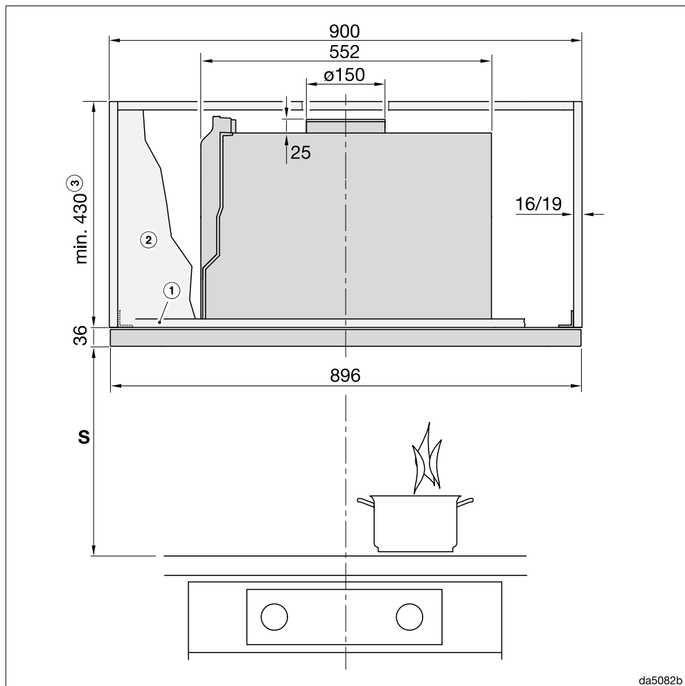
Rysunek 2: DAS 4930 w szafce o szerokości 900 mm.
