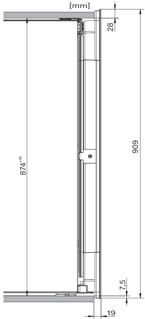
Näkymä sivulta
