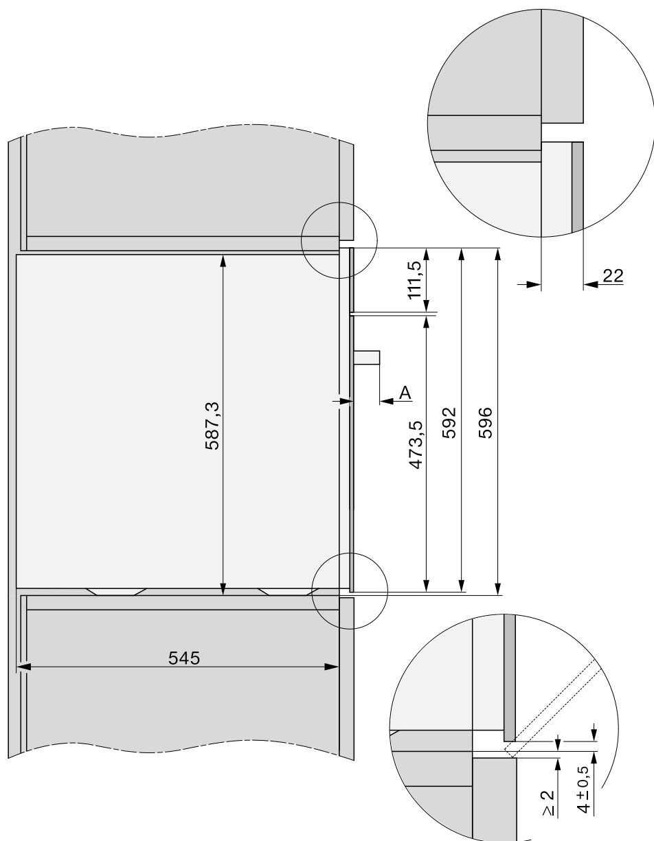
侧视图
