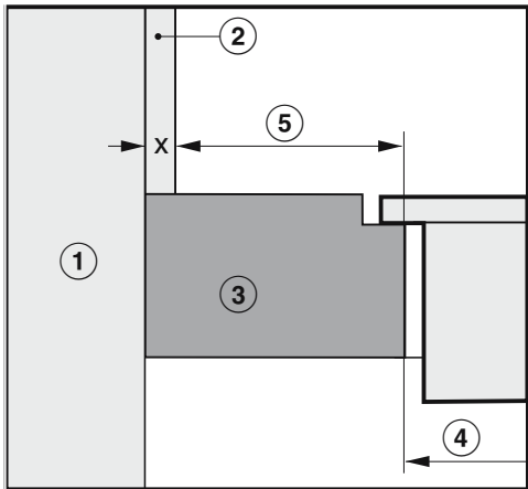
Flächenbündiger Einbau
