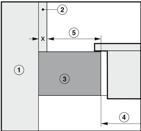
Aufliegender Einbau
