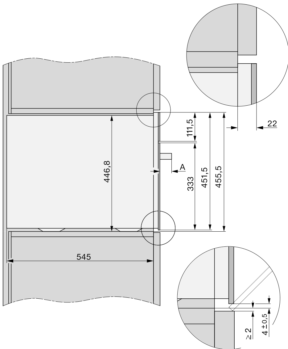
侧视图
