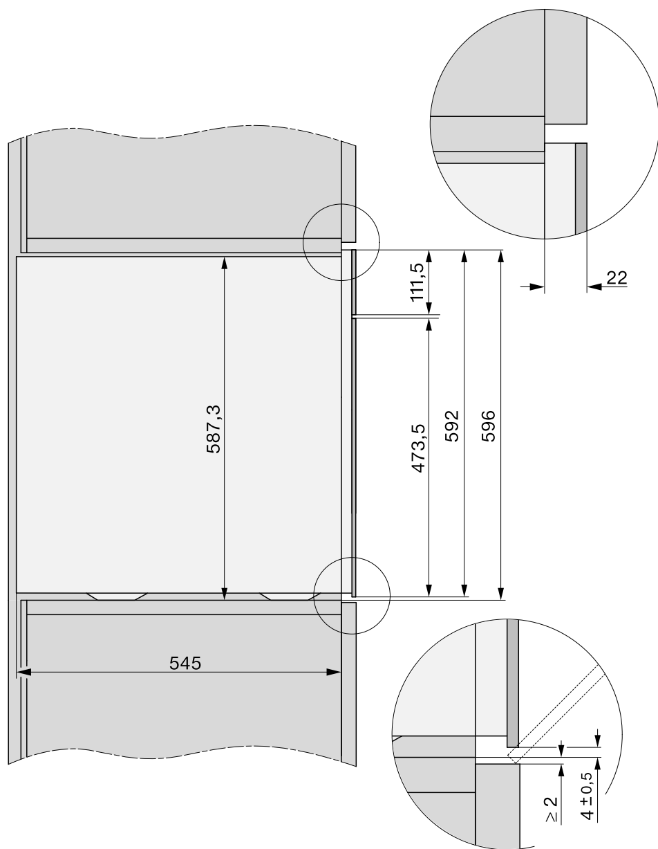
侧视图
