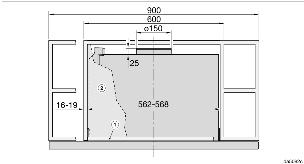
Bild 3: DAS 4931 in einem 600 mm breitem Schrank oder in einem 900 mm breitem Schrank mit seitlichen Fächern.
