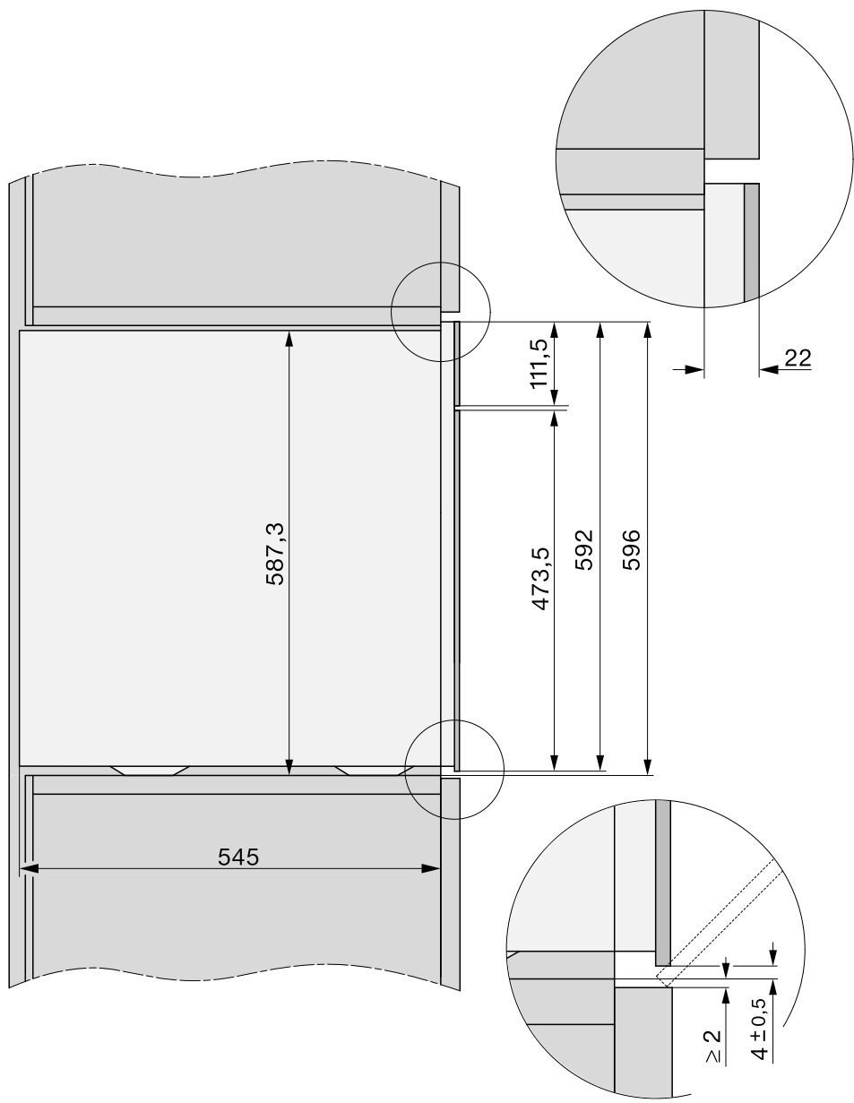
側視圖
