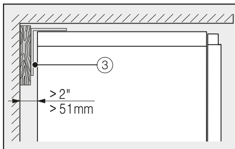
Fixation à un mur de béton
