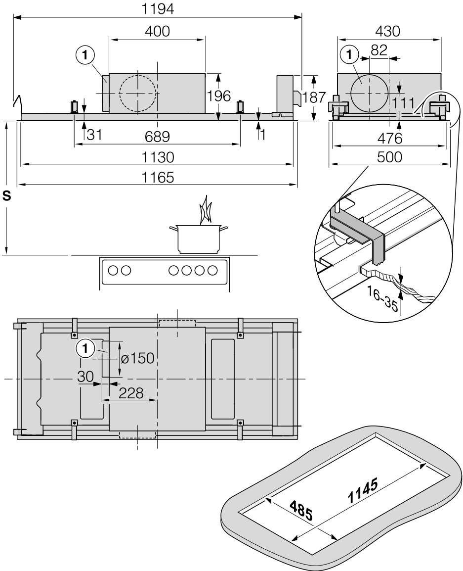
Baca bağlantılı işletimde DAC 2240
