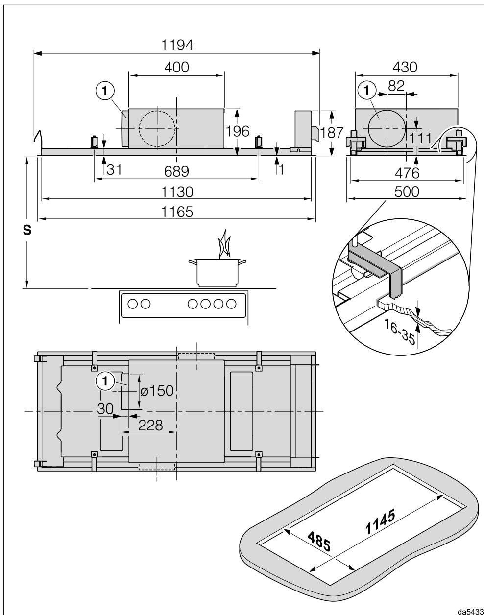
DAC 2240 en mode évacuation d'air
