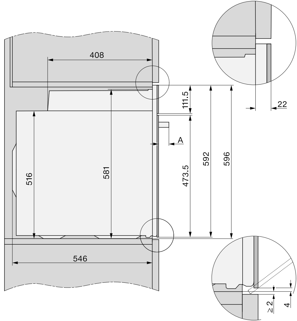
侧视图
