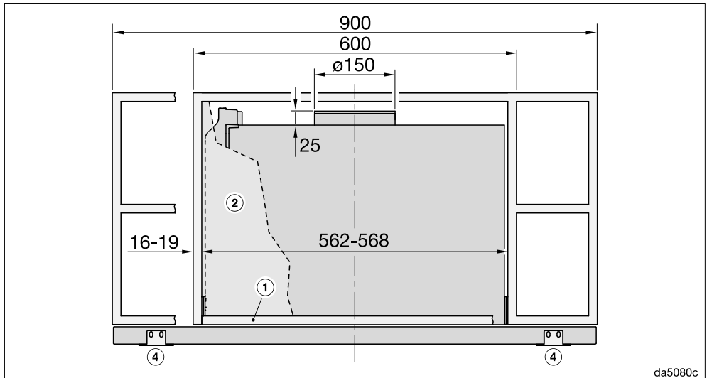
Bild 3: DAS 4920 in einem 600 mm breitem Schrank oder in einem 900 mm breitem Schrank mit seitlichen Fächern.
