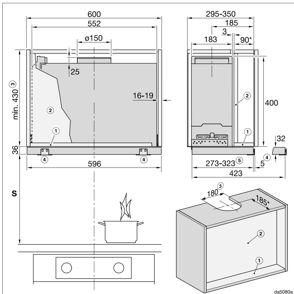
Rysunek 1: DAS 4620 w szafce o szerokości 600 mm.
