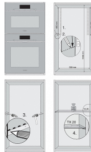
ENB1060, Kombination 45er + 60er Nische, Skizze
