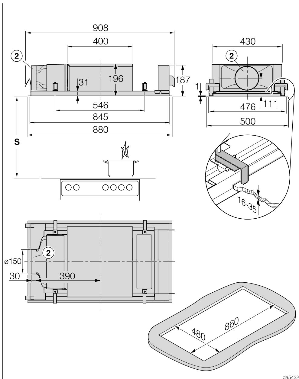
DAC 4940 en mode recyclage et recirculation Plug&Play
