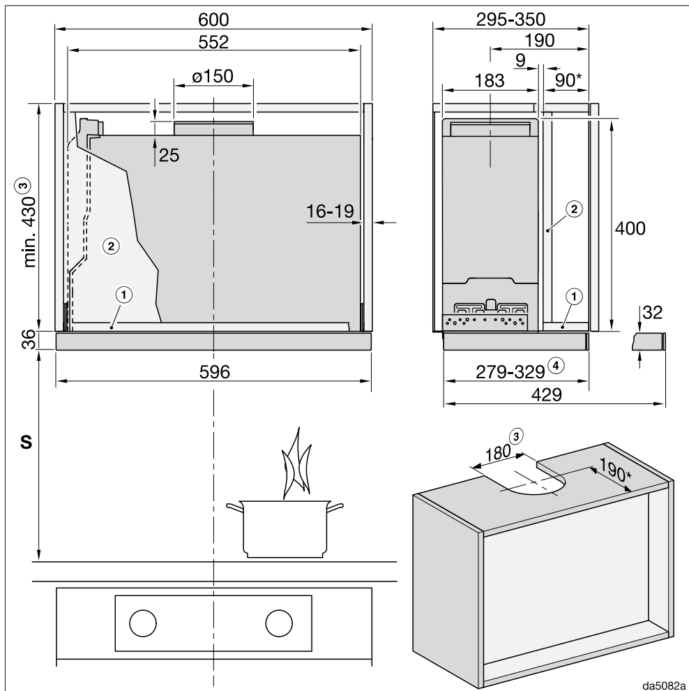
Bild 1: DAS 4630 in einem 600 mm breitem Schrank.
