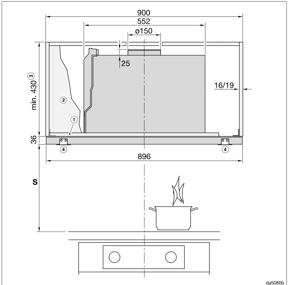
Bild 2: DAS 2922 in einem 900 mm breitem Schrank.
