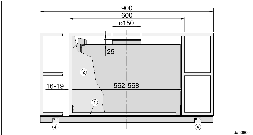
Bild 3: DAS 2922 in einem 600 mm breitem Schrank oder in einem 900 mm breitem Schrank mit seitlichen Fächern.
