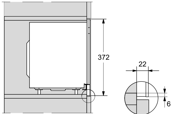
Zijaanzicht hoge kast
