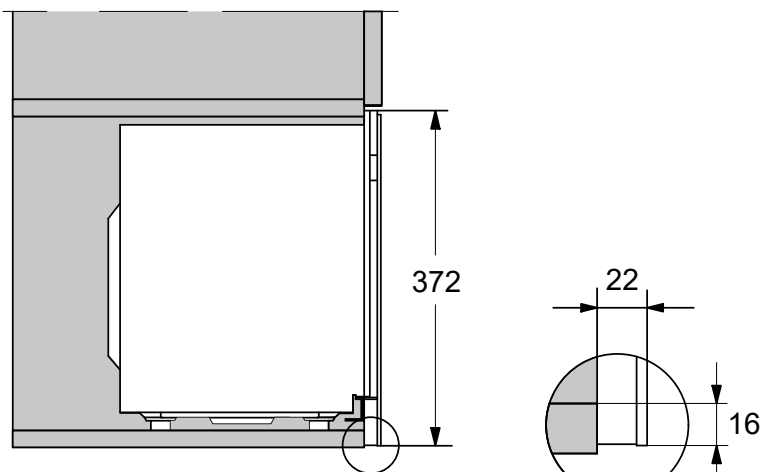
Zijaanzicht bovenkast
