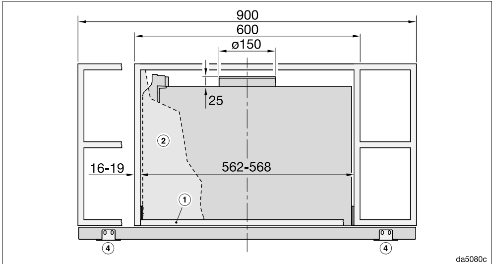
Bild 3: DAS 2922 in einem 600 mm breitem Schrank oder in einem 900 mm breitem Schrank mit seitlichen Fächern.
