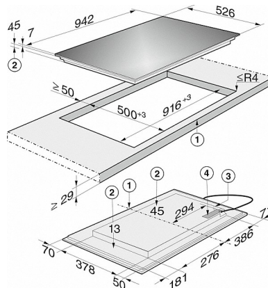
KM 6388 (skitse)
