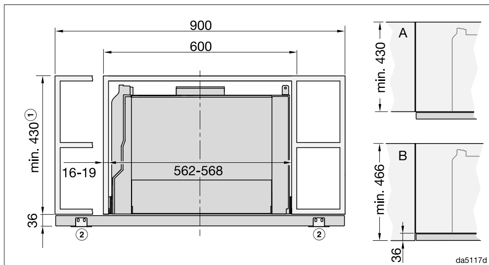
图 3: DAS 4920 安装在 900 毫米宽的橱柜中, 或者安装在带有侧隔间的 900 毫米宽的橱柜中
