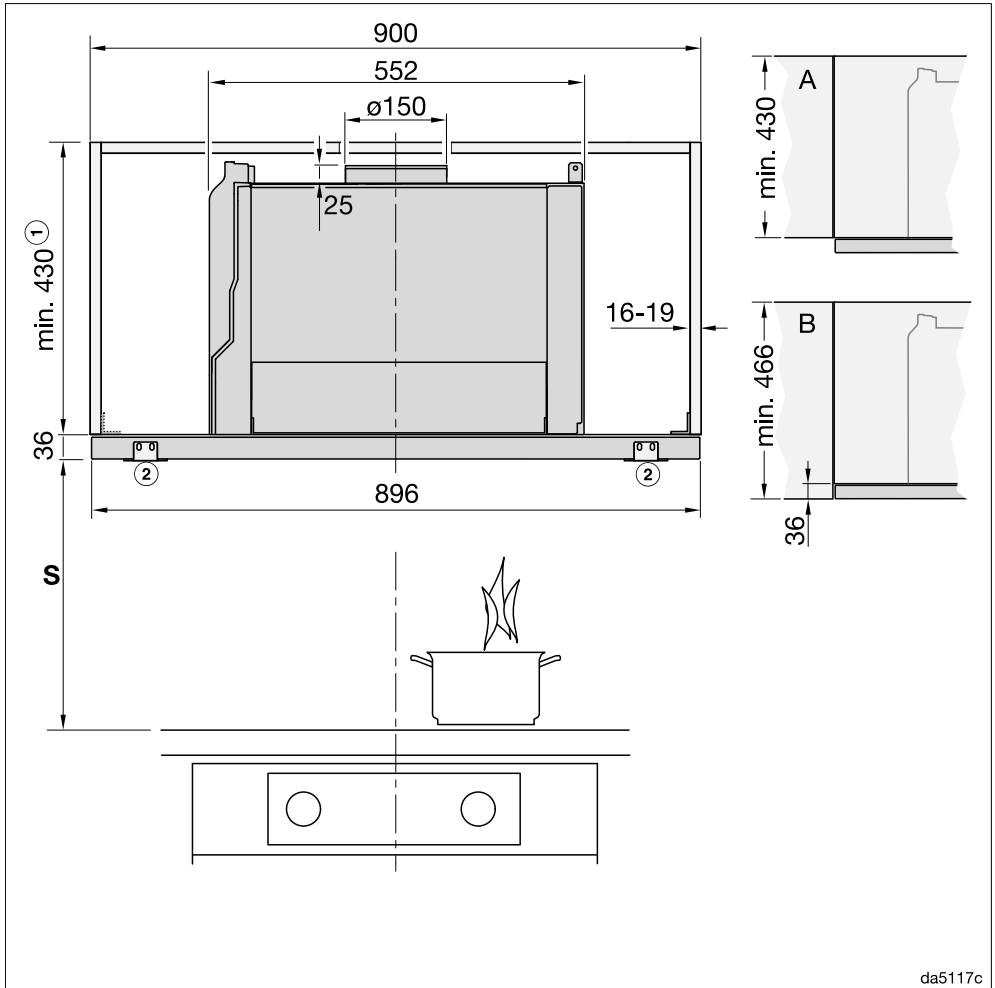
图 2: DAS 4920 安装在 900 毫米宽的橱柜中
