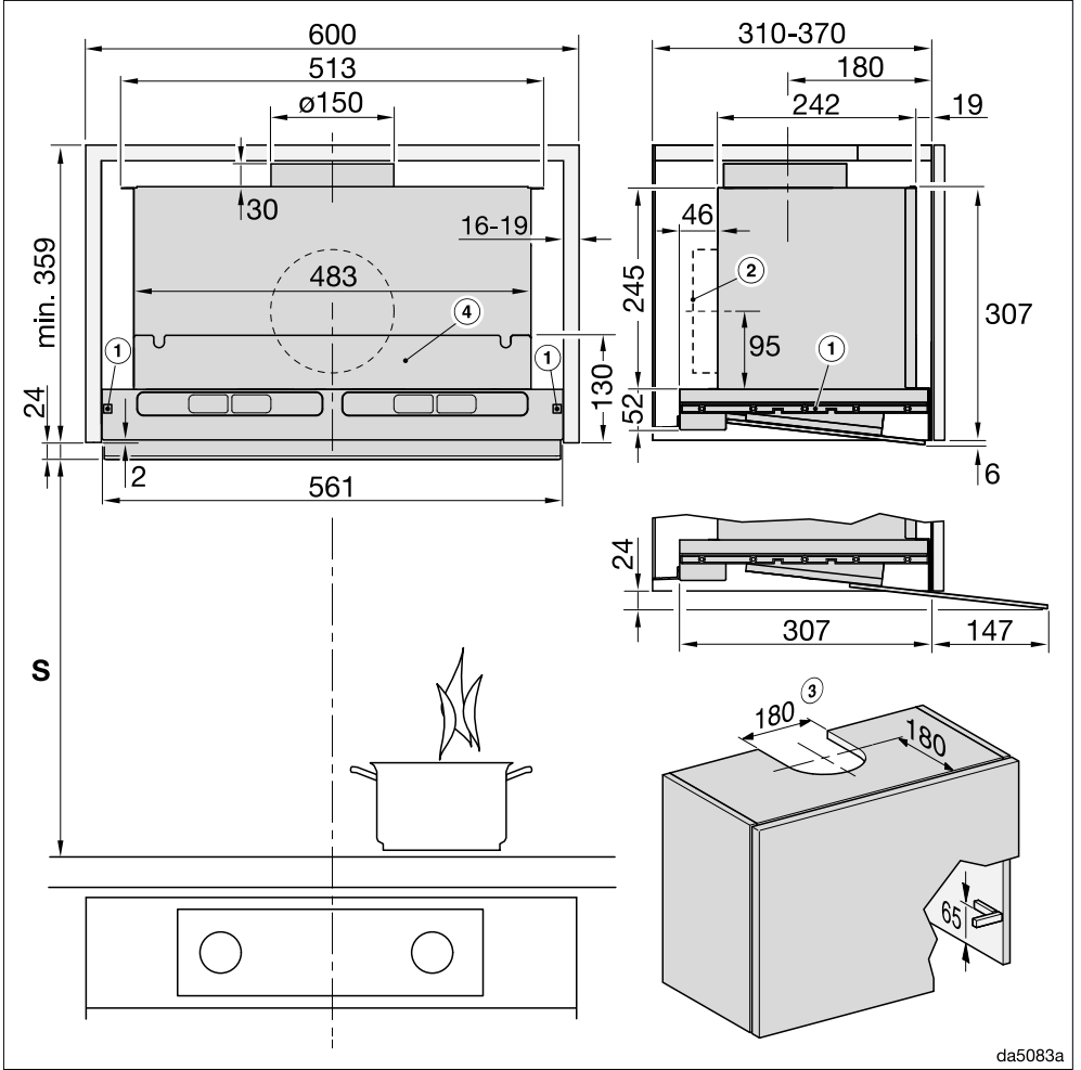
Resim 1: 600 mm genişliğinde bir dolap içinde DAS 4640.
