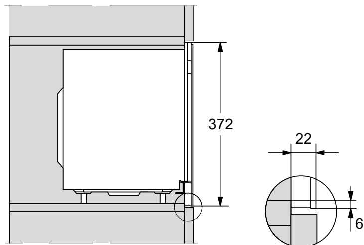
Widok z boku - szafka stojąca
