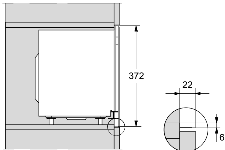
壁柜侧视图
