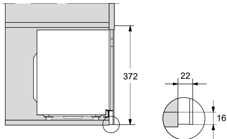
壁柜侧视图
