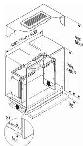
DAR 3000 (schéma)
