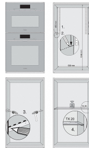
ENB 1060, combinatie 45-serie + 60-serie nis, schets
