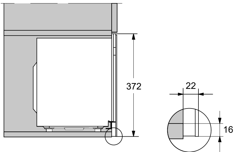
壁柜侧视图
